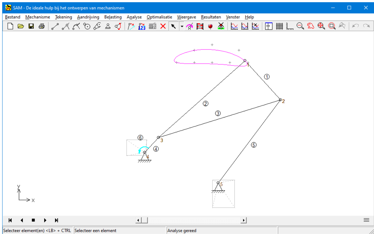
Handmatige trial&error oplossing + optimalisatiegebied van de gestelpunten
