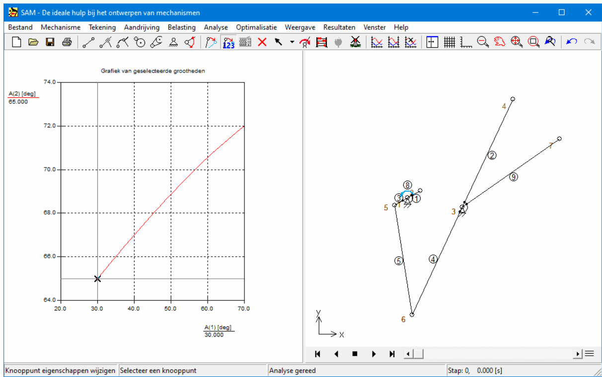
Resultaat van de (hoek)functiegeneratie (30 graden montagehoek van de slinger)
