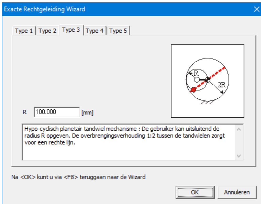
Exacte Rechtgeleiding : Hypocyclisch planetair tandwielmechanisme
