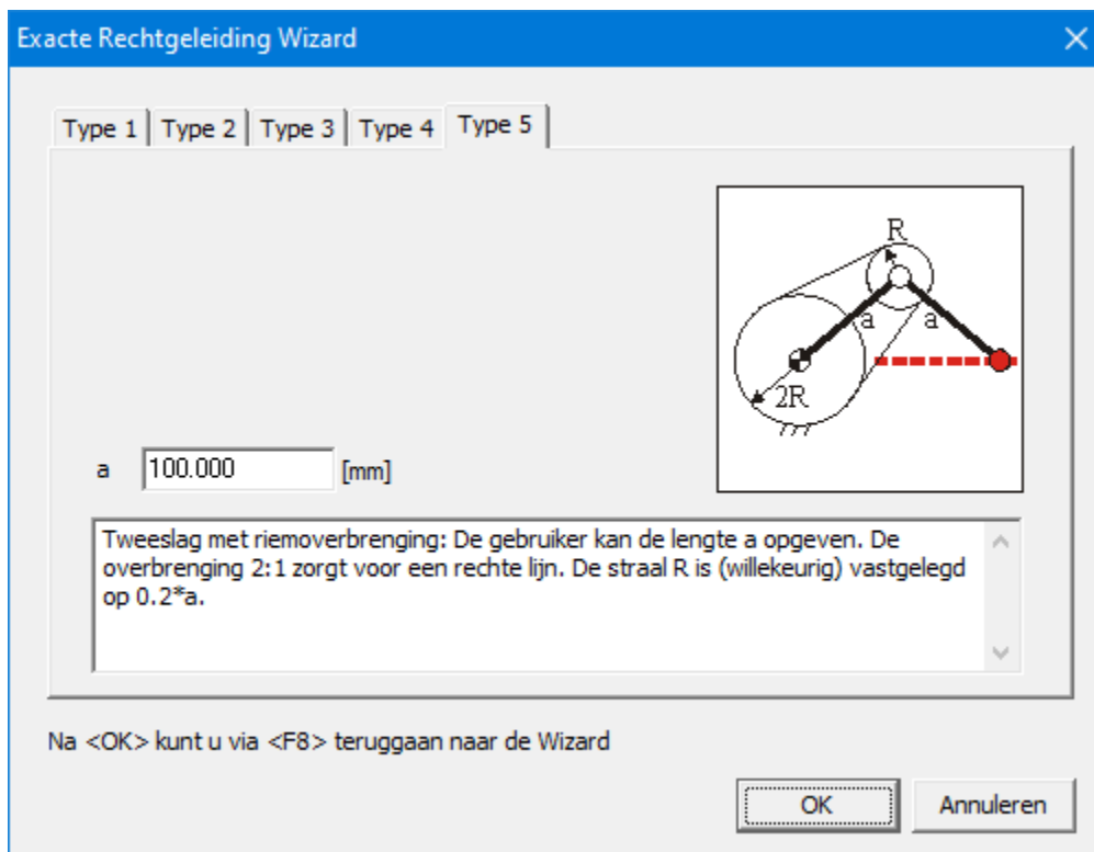
Exacte Rechtgeleiding : Tweeslag met riemoverbrenging
