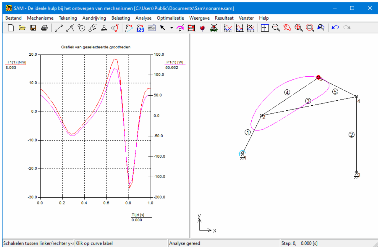
SAM 7.0 resultaten: Koppel (links) & Vermogen (rechts) in element 1 bij knooppunt
