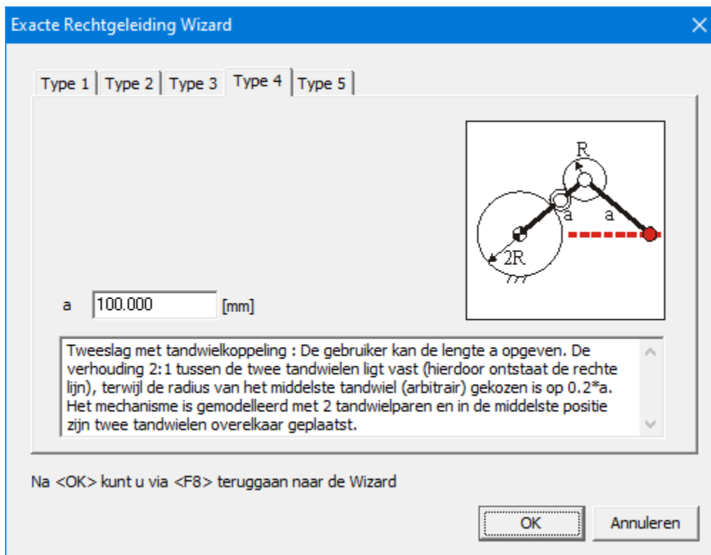
Exacte Rechtgeleiding : Tweeslag met tandwielkoppeling
