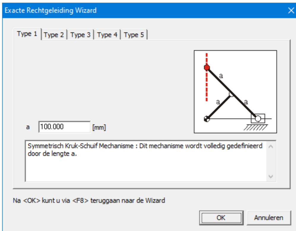
Exacte Rechtgeleiding : Symmetrisch kruk-schuif mechanisme
