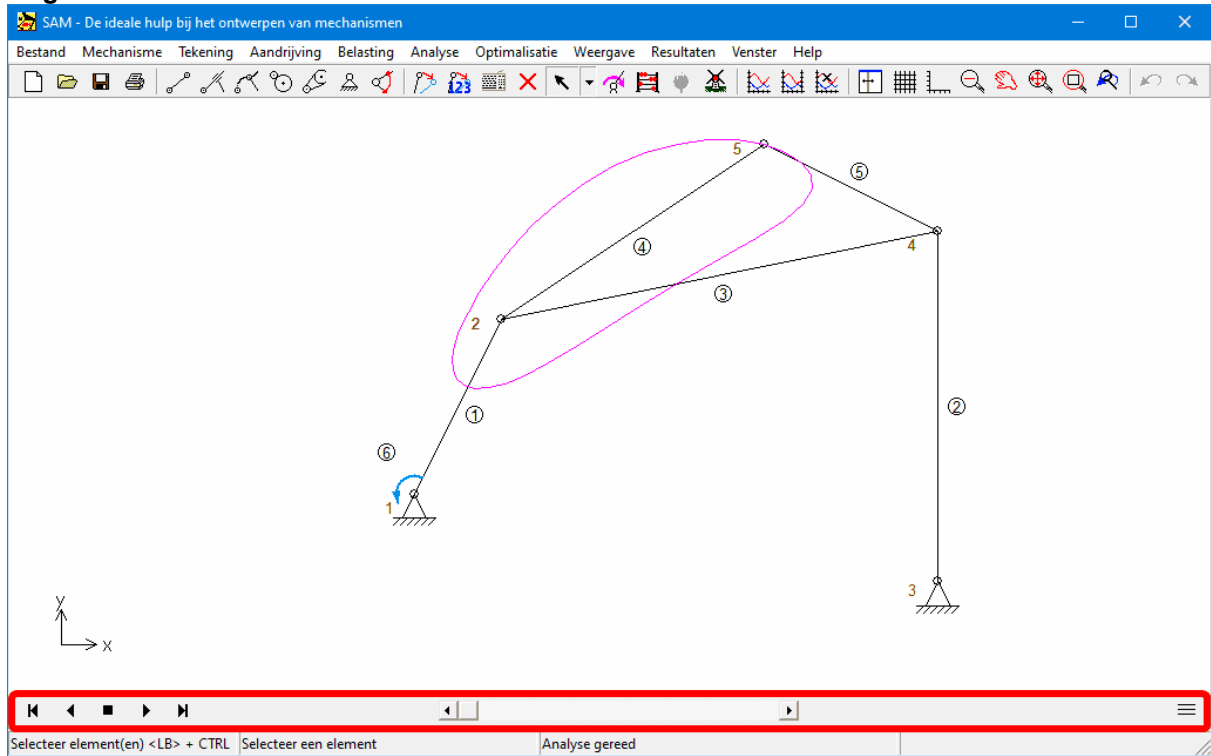
Screenshot met de nieuwe animatiefunctie
