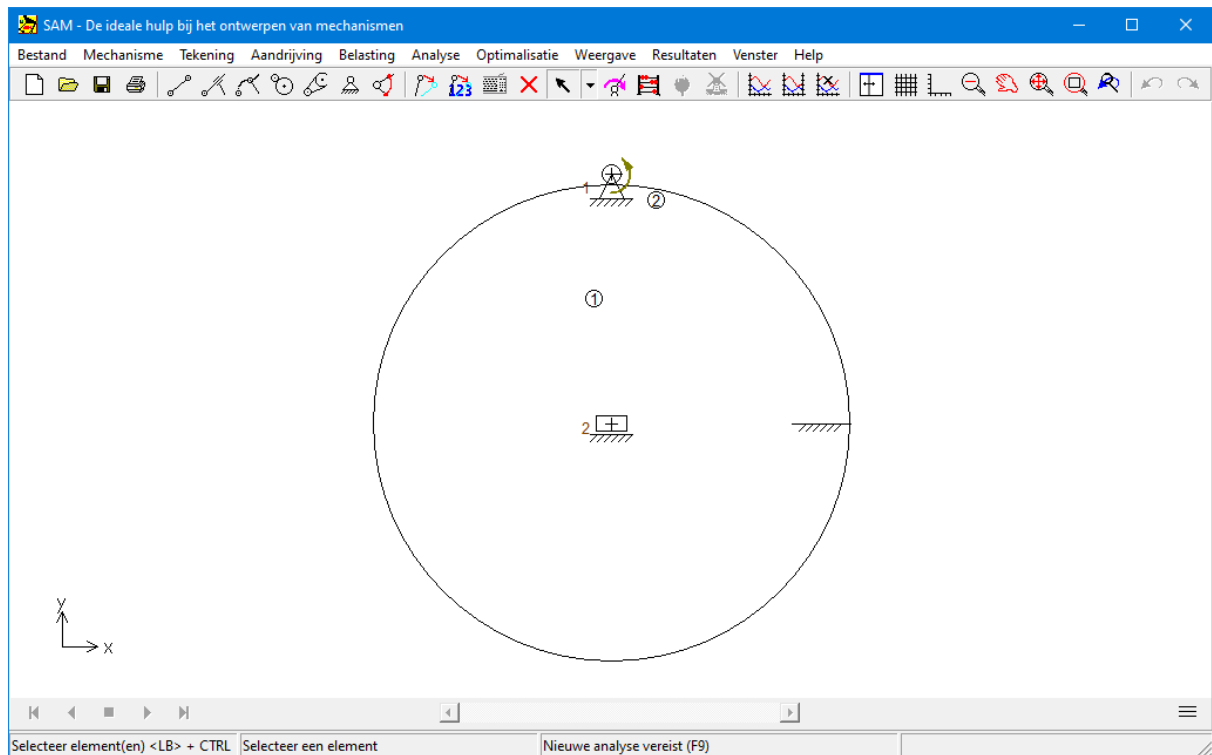
Simulatie van een tandheugel op basis van het tandwiel-element (RACK1.SAM)
