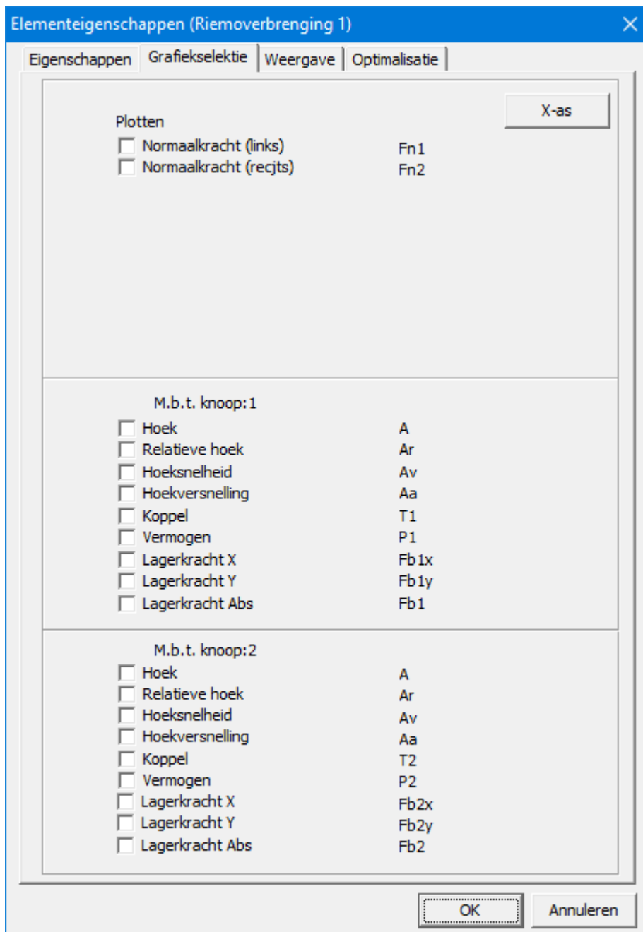
Berekenbare grootheden van een riemoverbrenging
