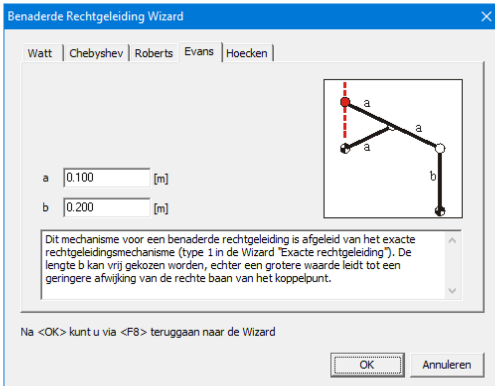
Benaderde Rechtgeleiding : Evans
