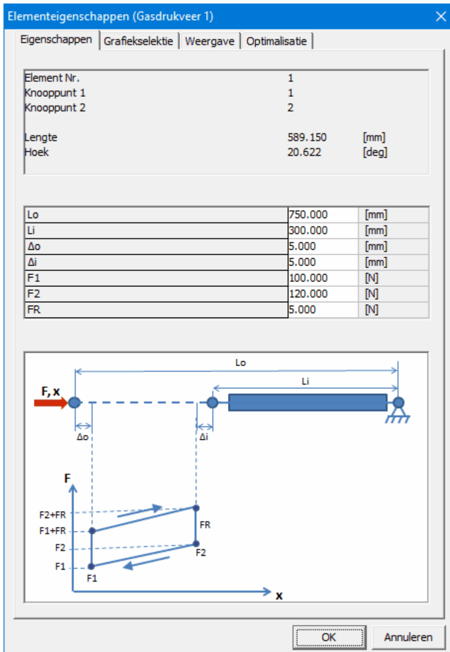
Element dialoog van de nieuwe gasdrukveer
