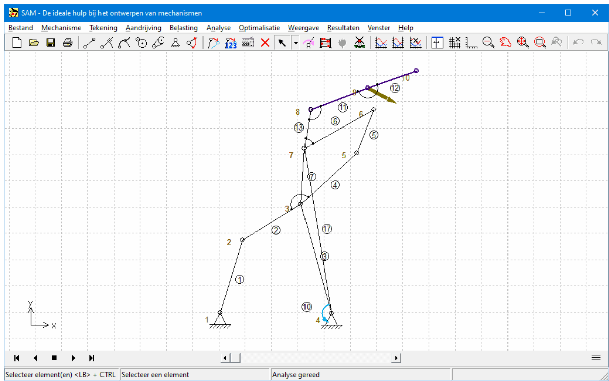
Spoiler mechanisme met kracht op knooppunt 9 (SCS.SAM)
