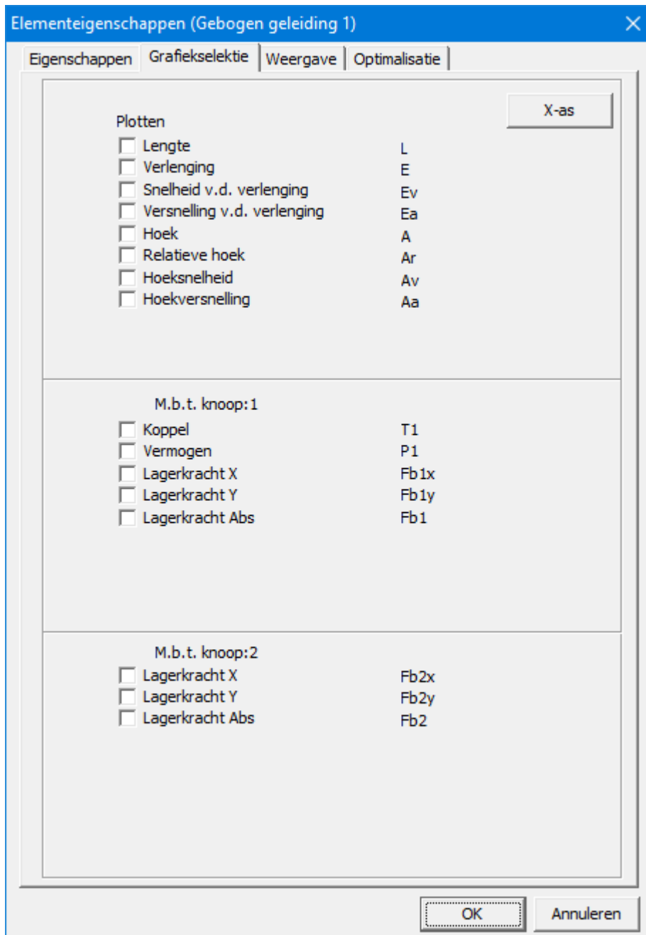
Resultaten van een gebogen geleiding
