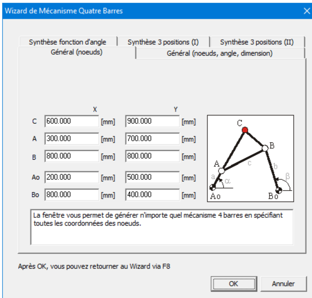
Wizard de conception de Mécanisme à 4 barres : Général (nœuds)
