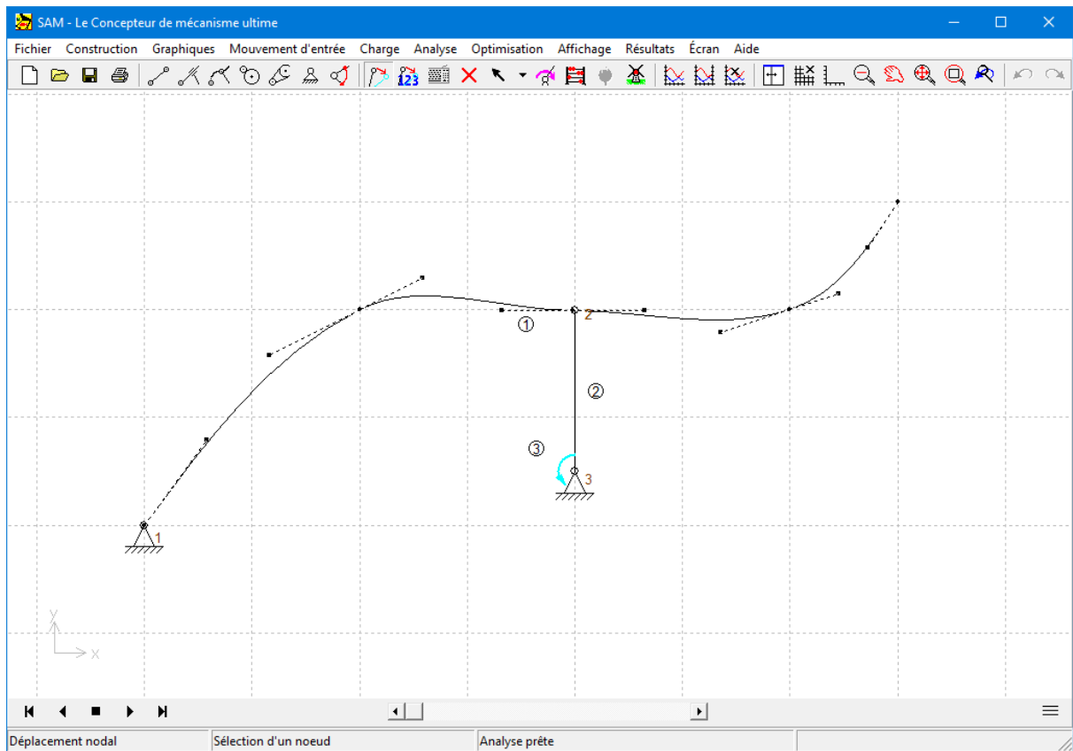
La définition de l'élément guidage courbe est basée sur les points de Bézier
