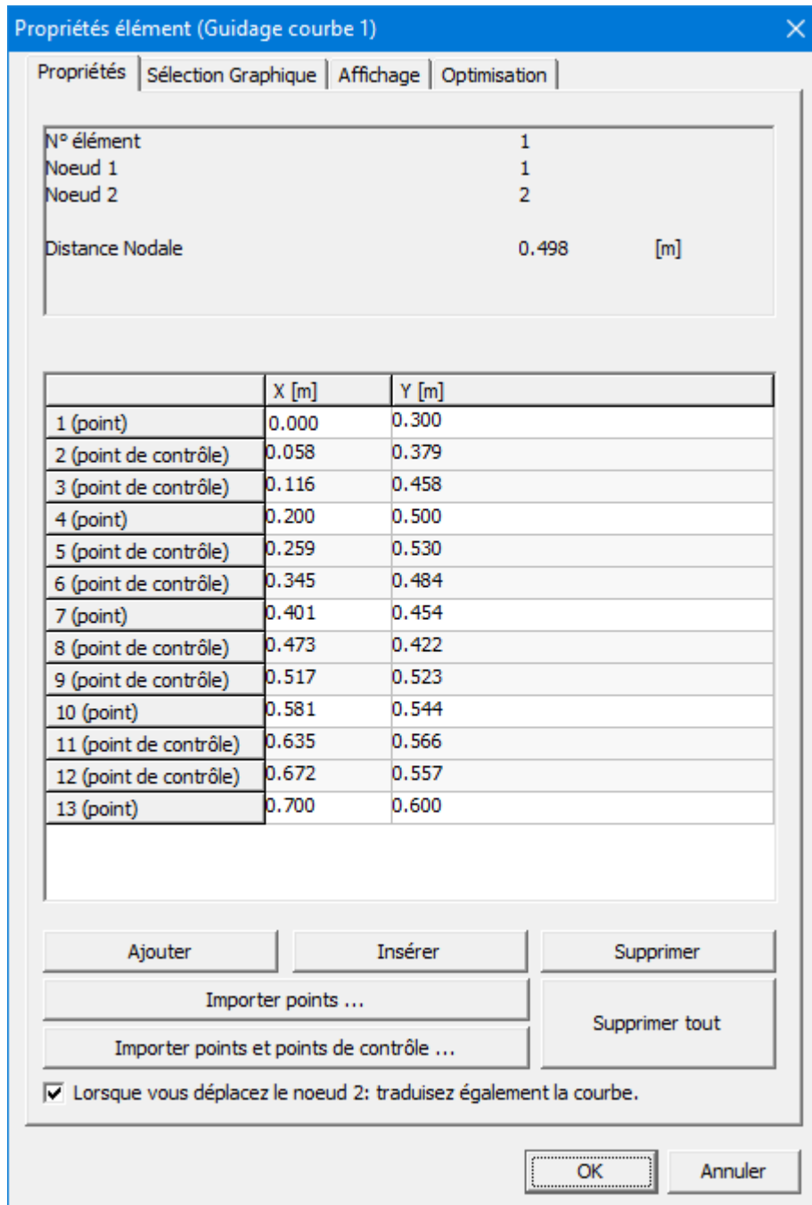
Propriétés de l'élément guidage courbe
