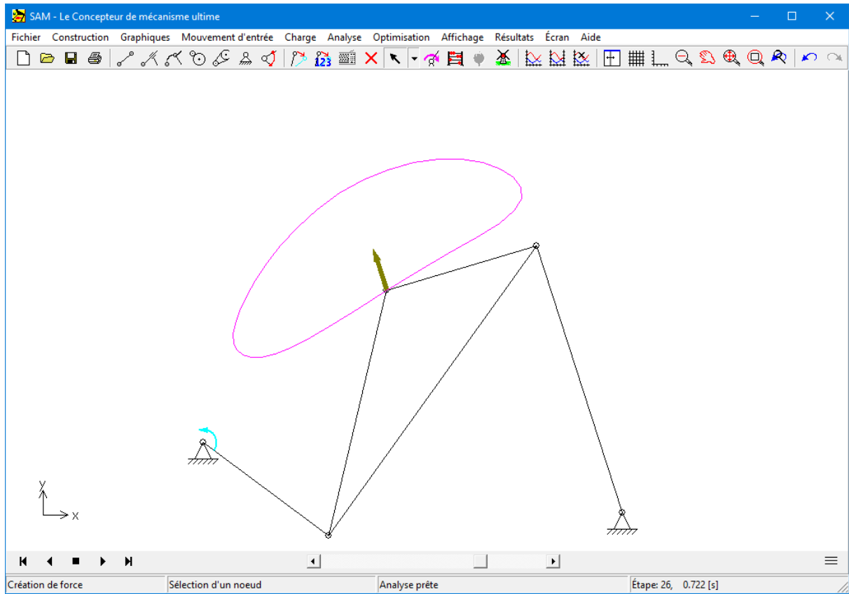
Exemple: force de 500 N sur le noeud 5 avec une direction identique à l'angle de l'élément 2)
