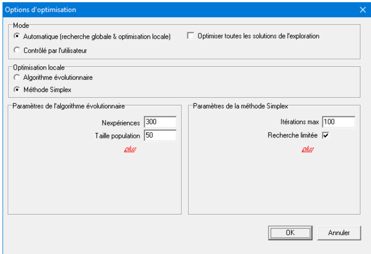
Fenêtre d'options d'optimisation standard
