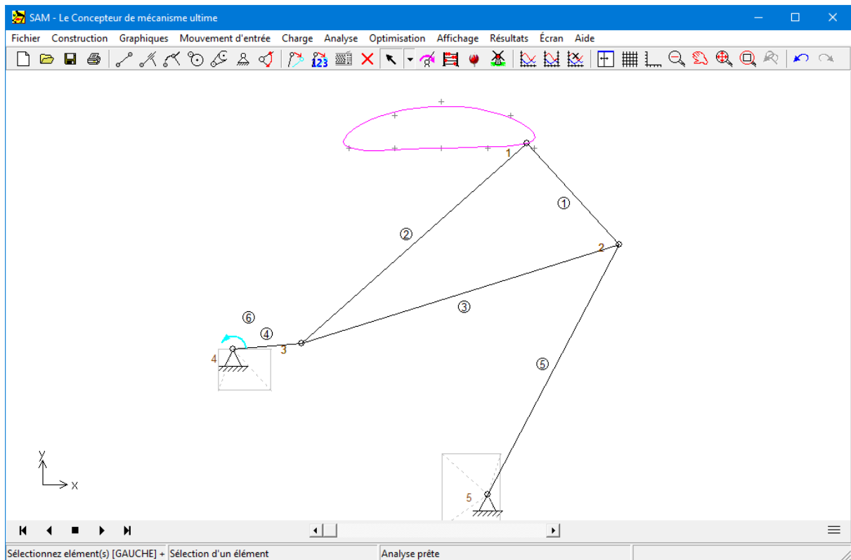
Mécanisme à 4 barres optimisé
