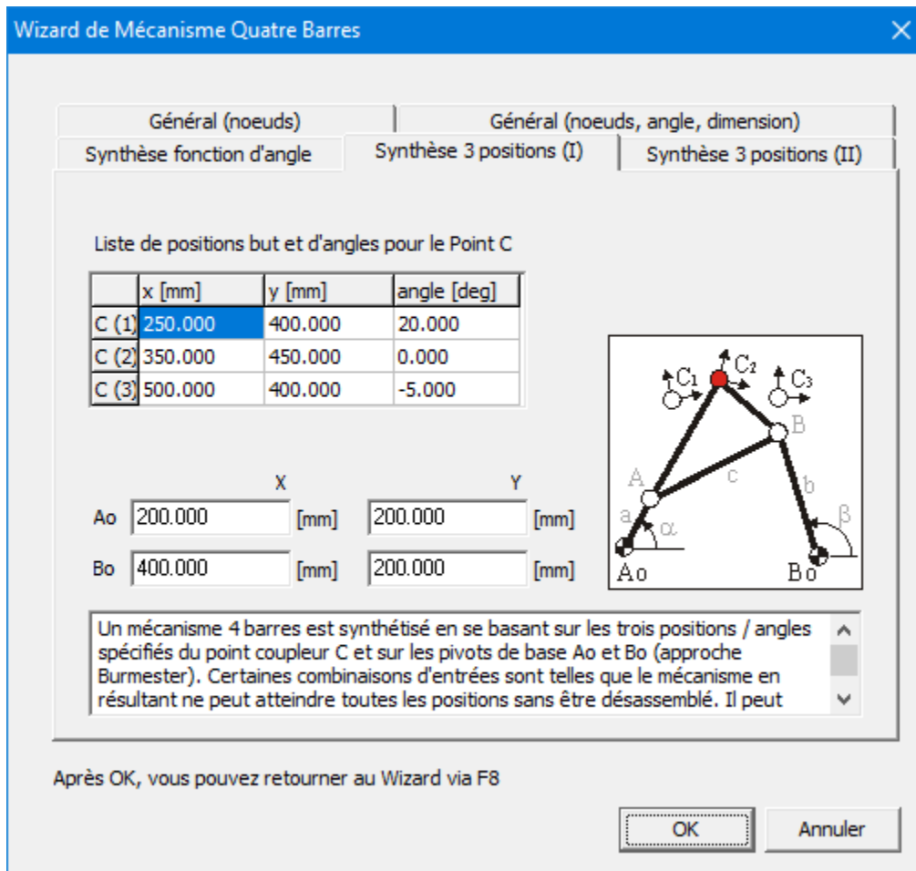
Wizard de Mécanisme à 4 barres : Synthèse 3 positions (I)
