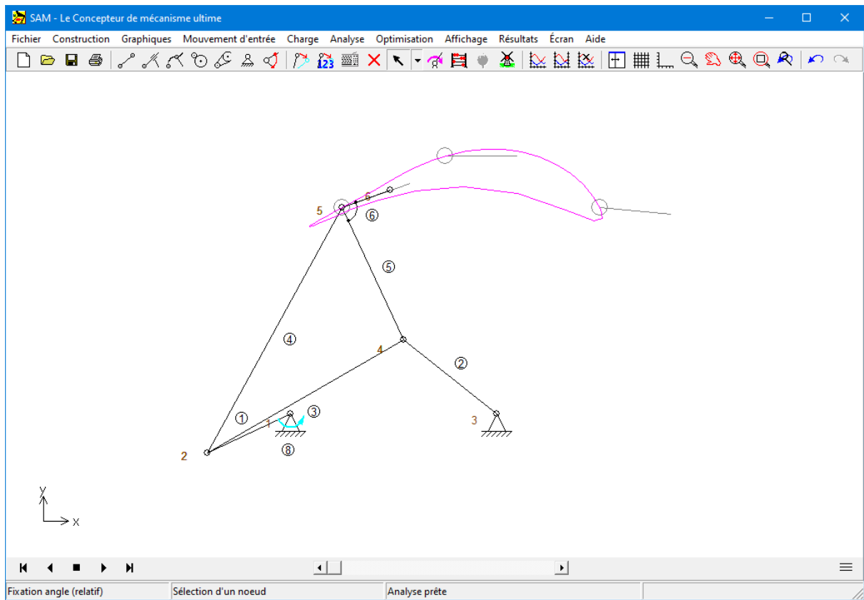
Mécanisme à 4 barres synthétisé incluant les trois positions / angles prescrits du point coupleur.
