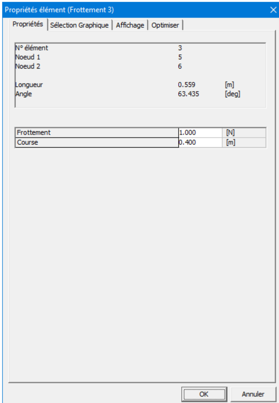
Propriétés de l'élément frottement
