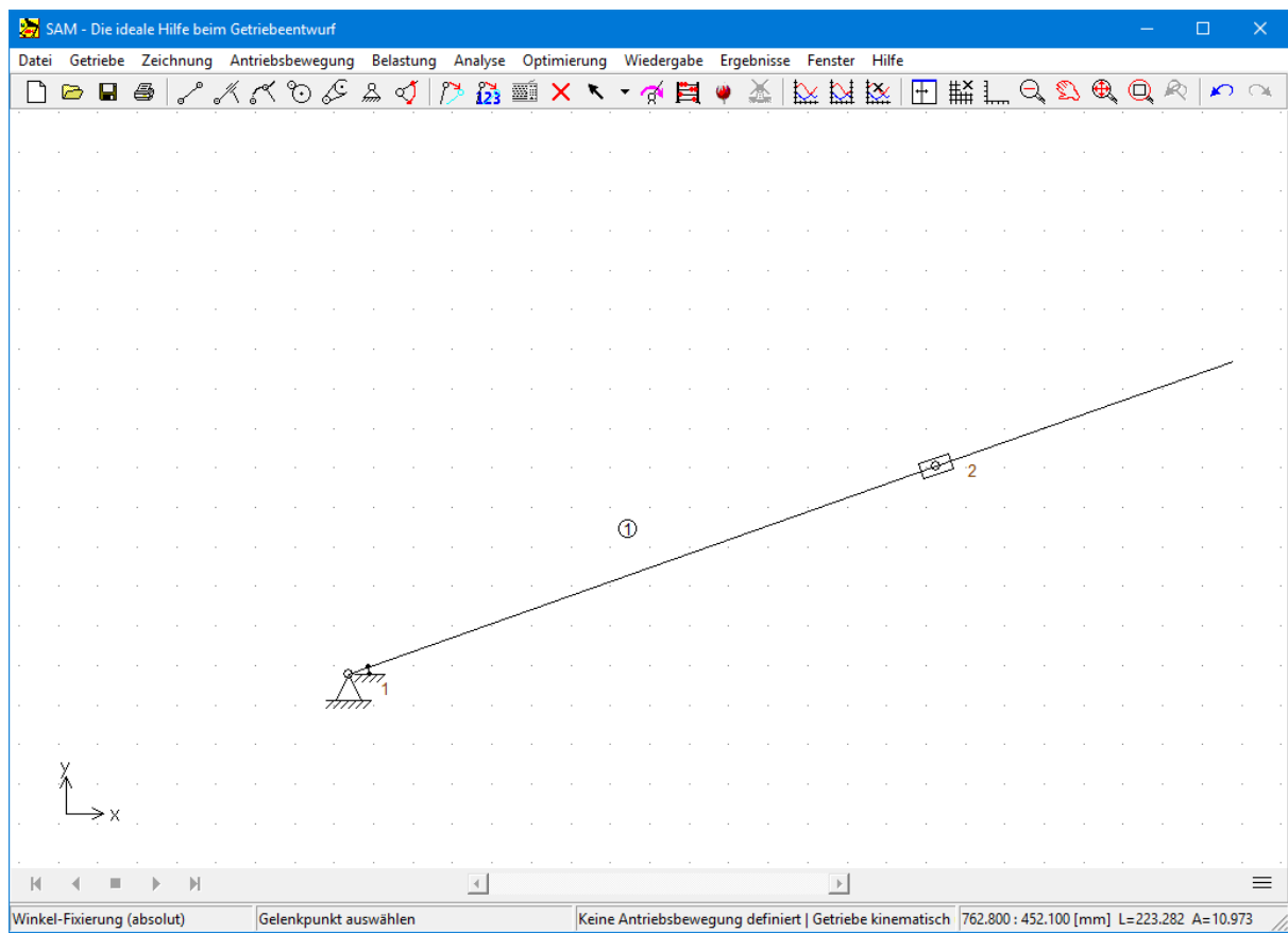
Erstellen einer geneigten Geradföhrung mit Verwendung eines Schubgelenkes
