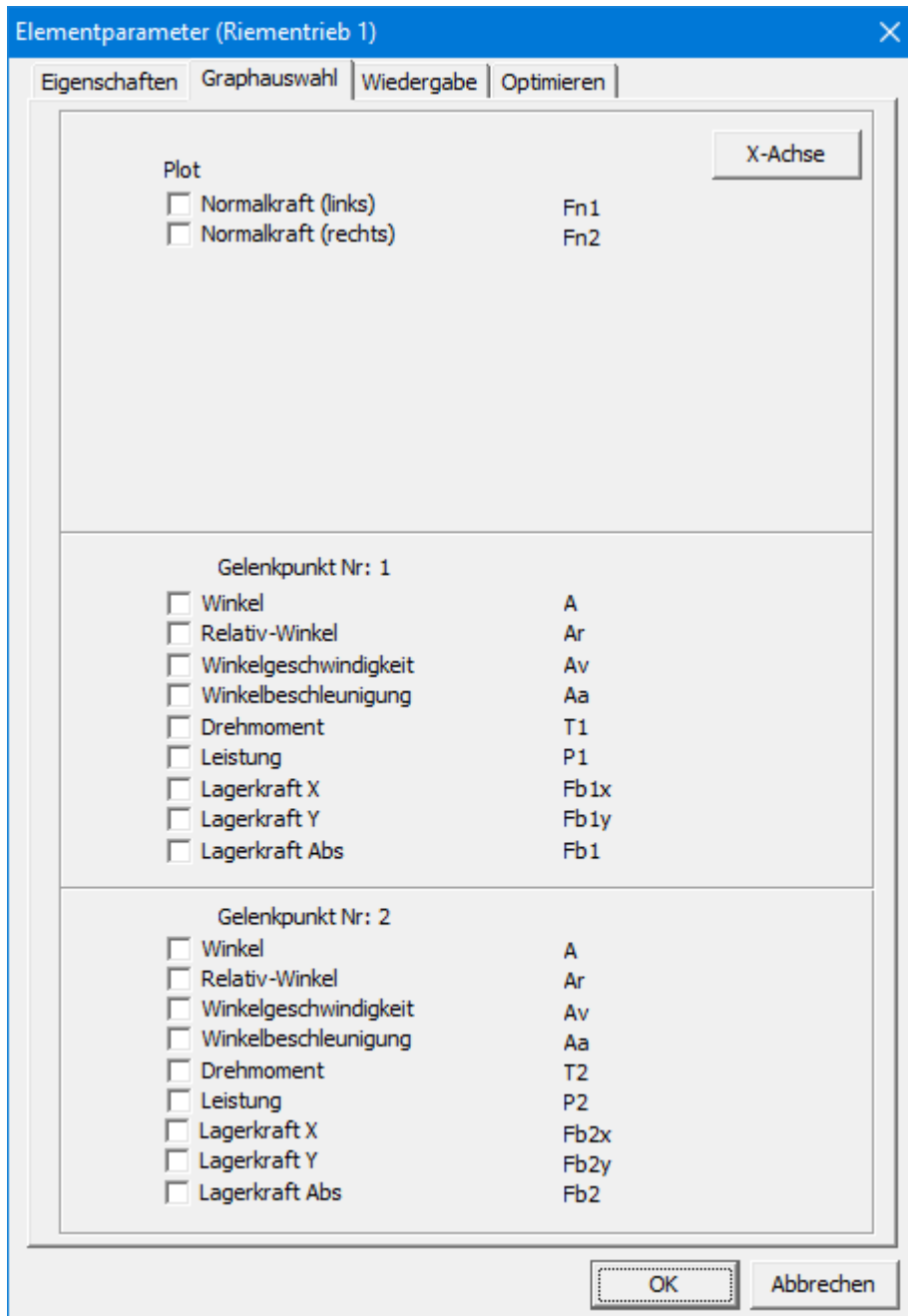
Berechenbare Eigenschaften eines Riementriebes
