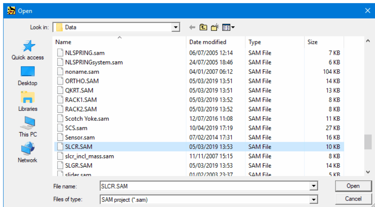
Datei/Laden Dialogfenster
