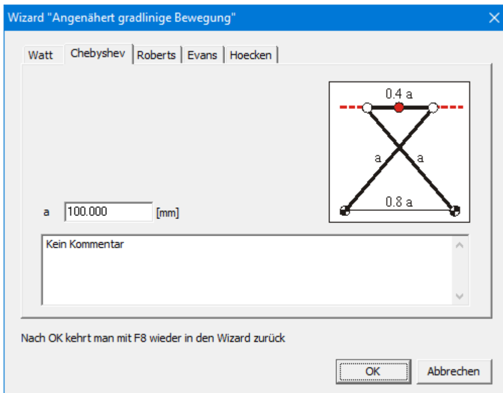
Design Wizard Angenäherte Geradführung "Chebyshev"
