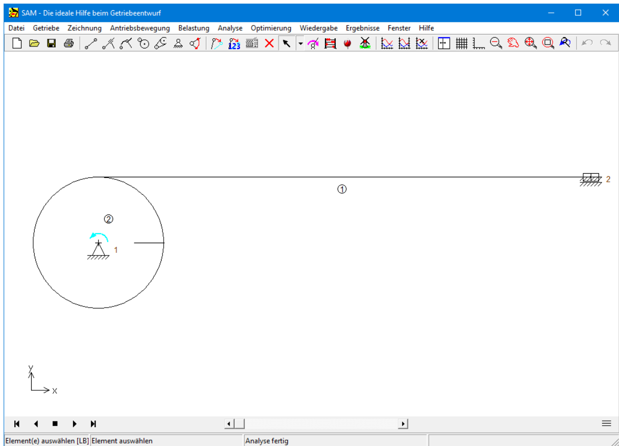
Modellierung einer Zahnrad/Zahnstange mittels Riemen-Element (RACK2.SAM)
